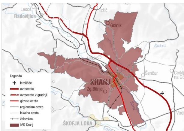
Karta 7 Prometna infrastruktura na območju MO Kranj
