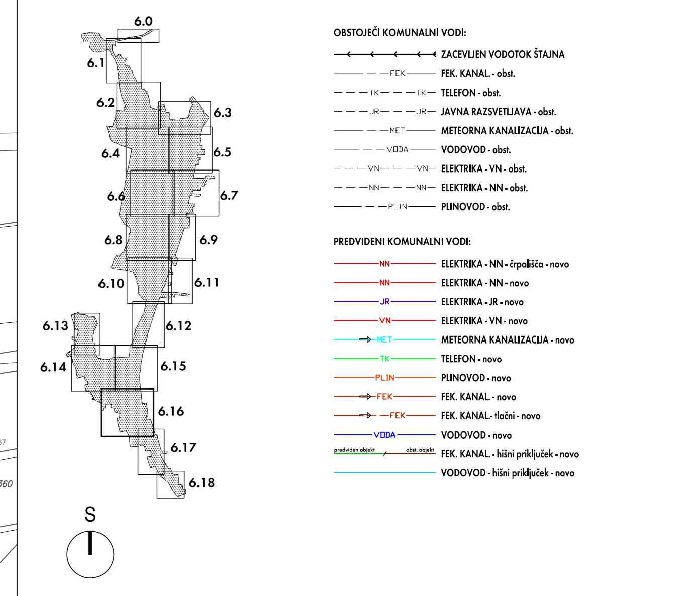
ZBIRNA SITUACIJA KOMUNALNIH VODOV M 1:500
